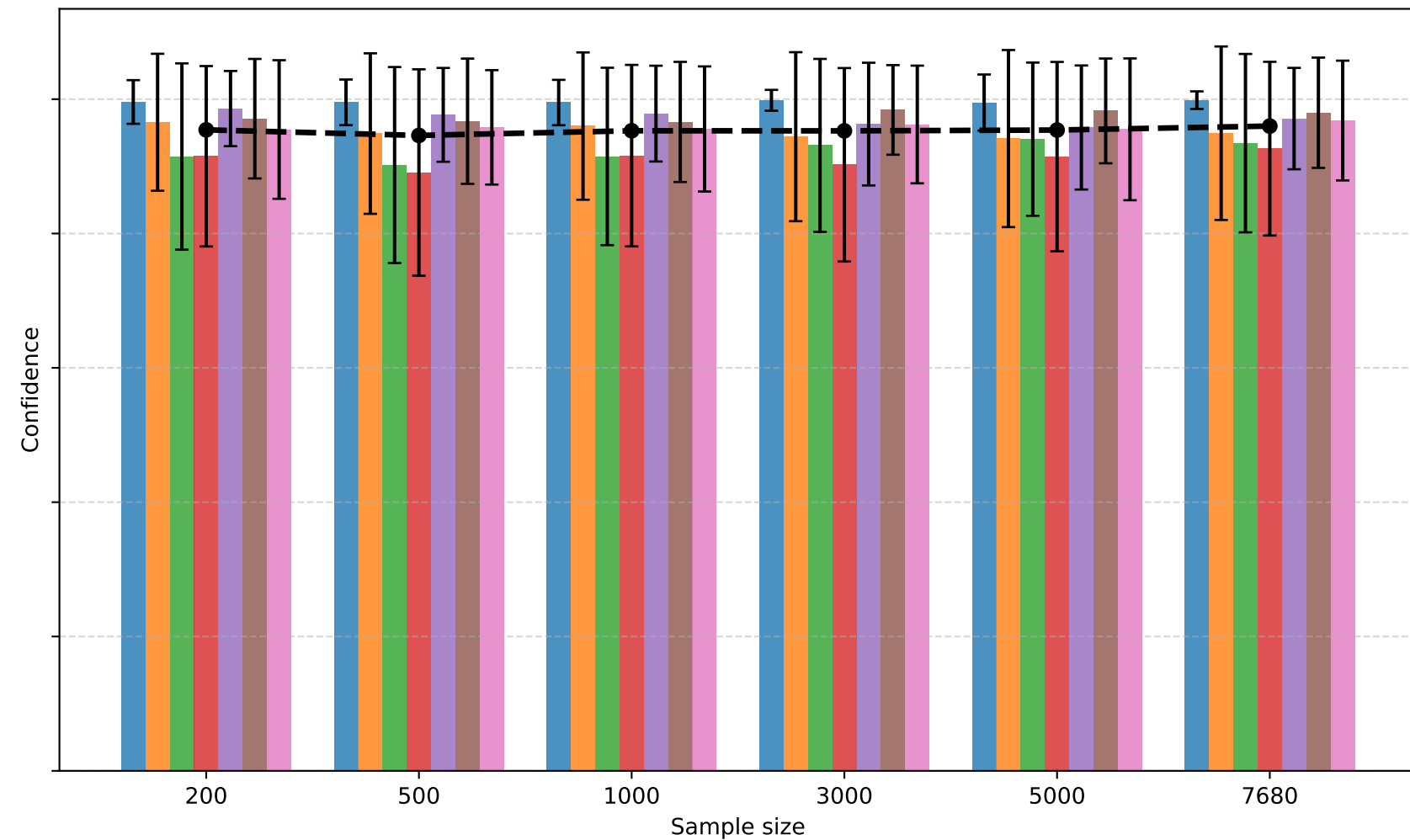
RDA
