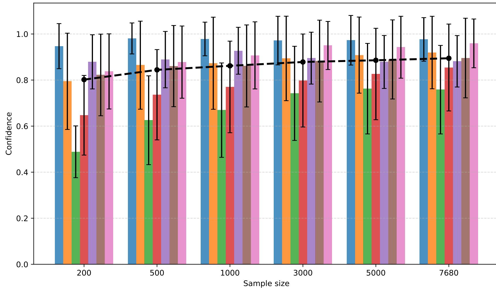
KNN
