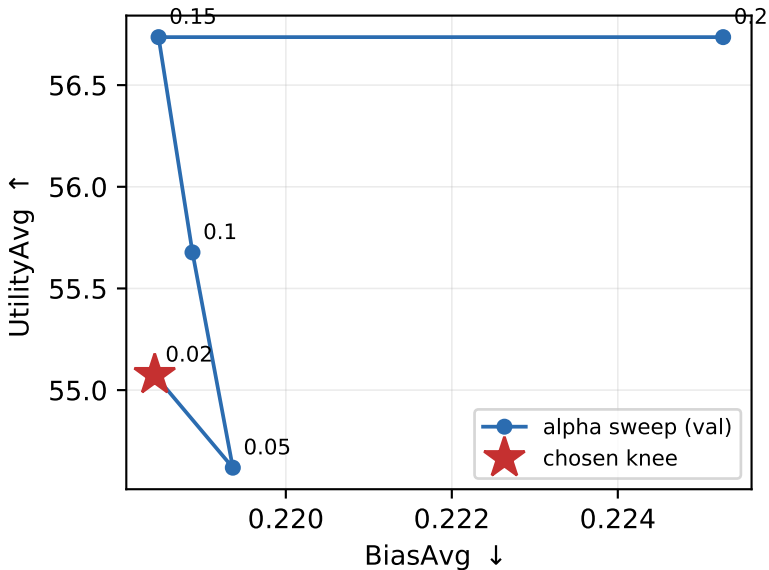
Ablation: \alpha -- LLaMA-2-13B
