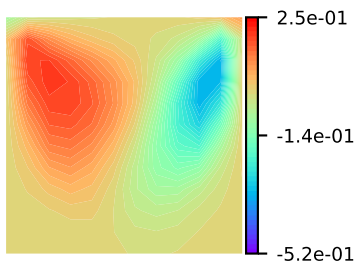
\hat{v}(x)
