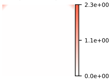
|p(x) - \hat{p}(x)|
