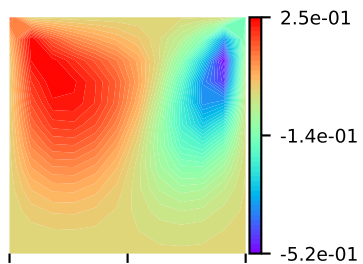
v(x)
