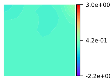
\tilde{p}(x)
