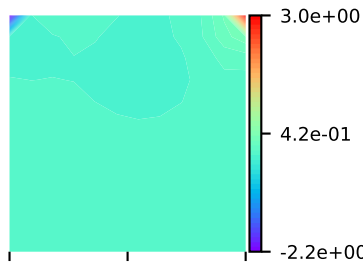
p(x)
