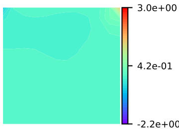
\hat{p}(x)
