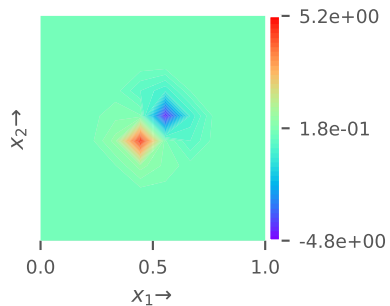
f(x)
