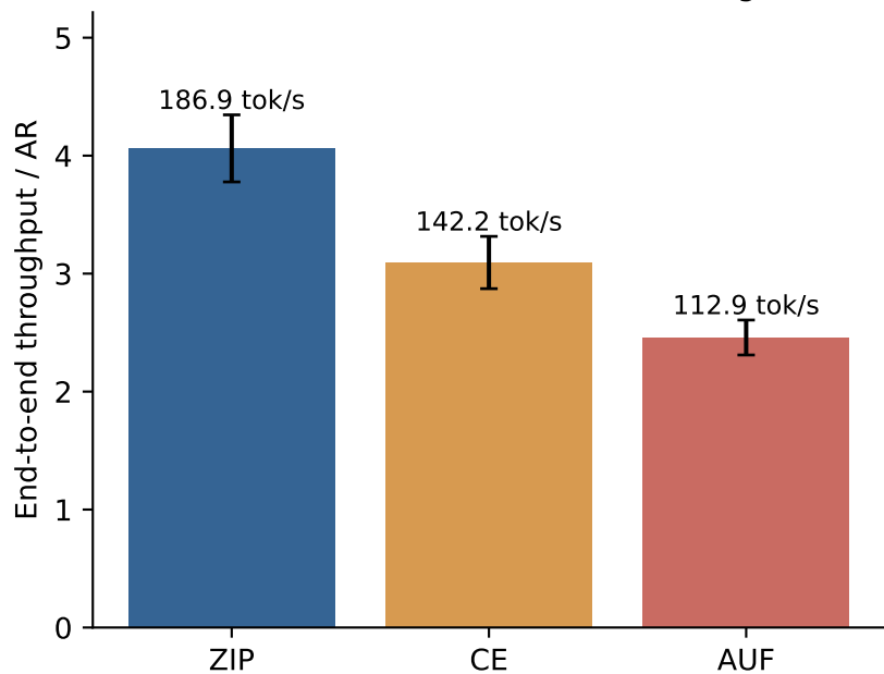
Llama: 3.1-8B drafter → 3.2-3B target
