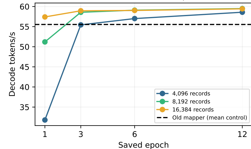
Qwen → Llama: zip
