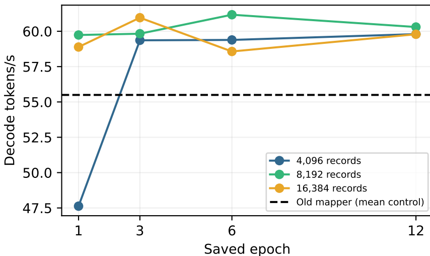
Qwen → Llama: dense
