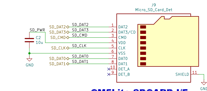
CM5Lite SDCARD I/F
