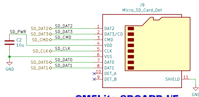
CM5Lite SDCARD I/F
