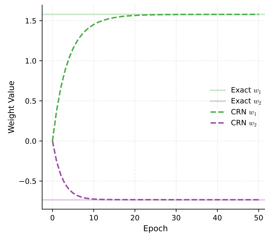
Parameter Evolution (Weights)
