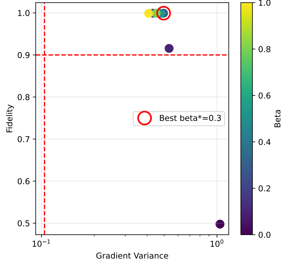
Pareto Frontier
