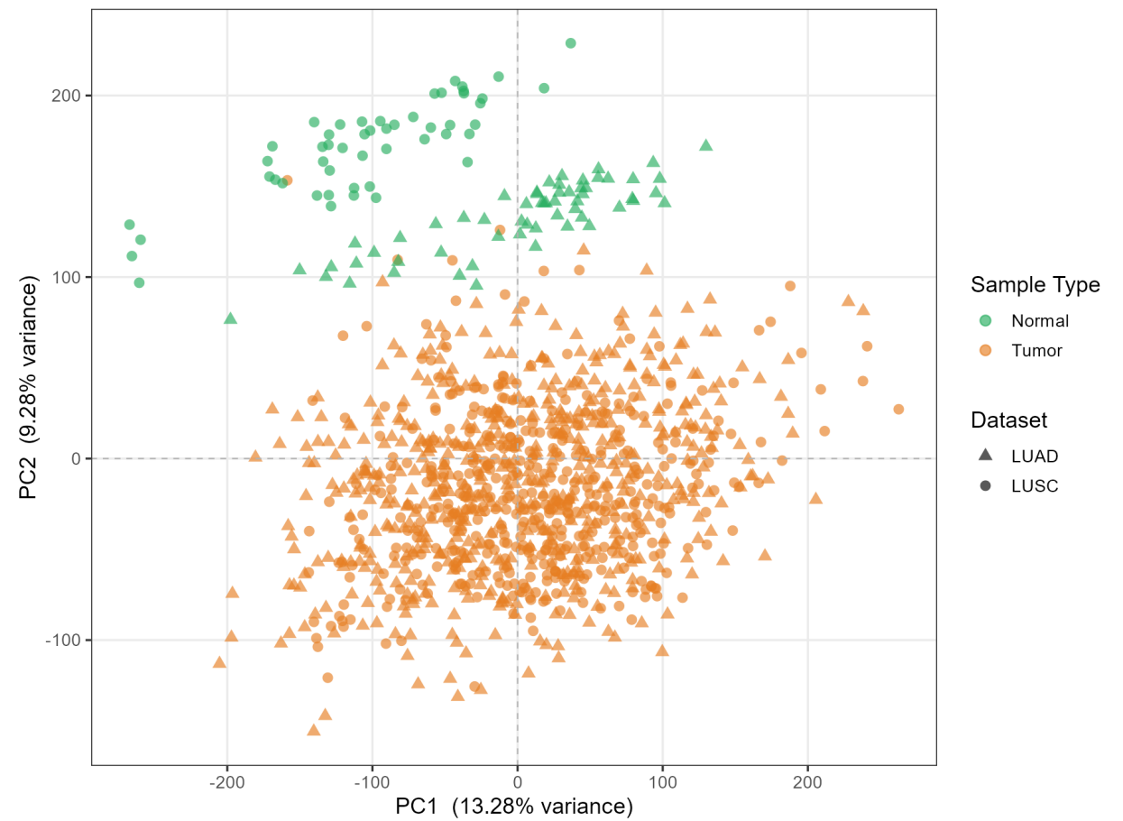
Final PCA — Tumor vs Normal
