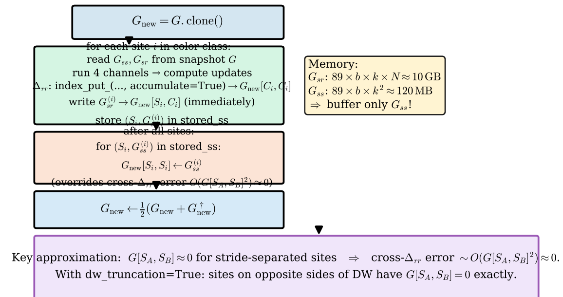
(d) GPU write-back — deferred G_{ss} to save memory
