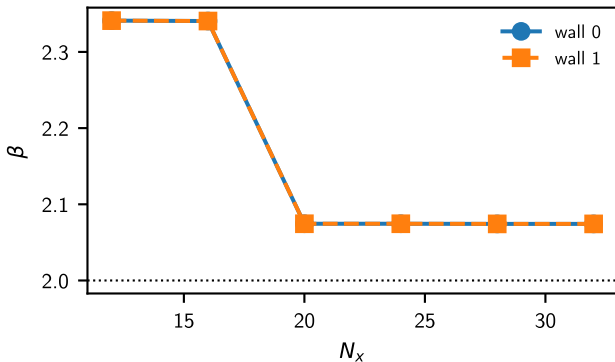
hard_exterior: wall correlator
