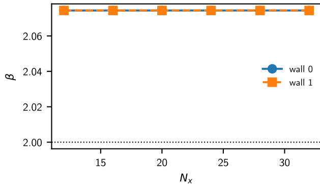
hard_exterior: wall correlator
