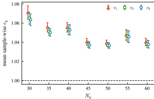
(c) Cardy--Calabrese conversion; error: SEM
