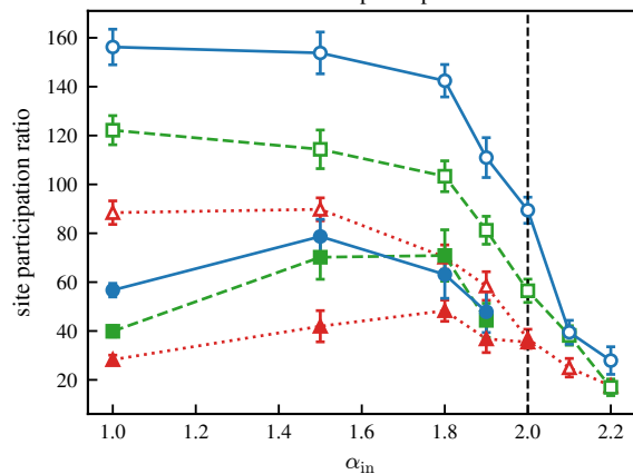
finite-mode participation
