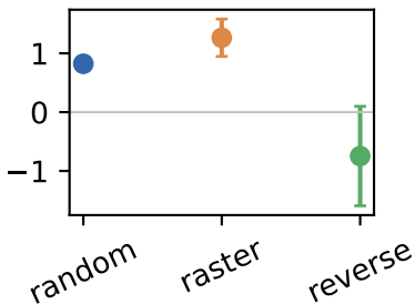
v left
