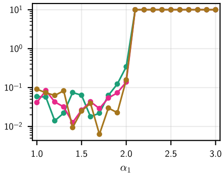
NaN \rightarrow 10
