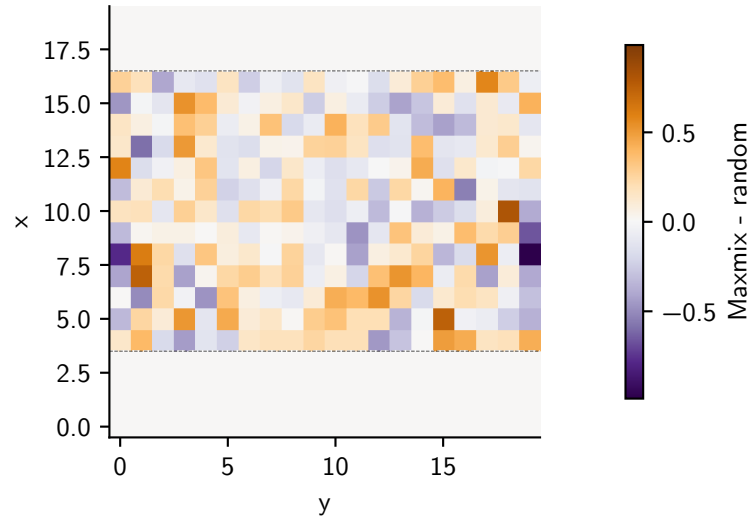
DW alpha=1/30, dwtrunc=1
