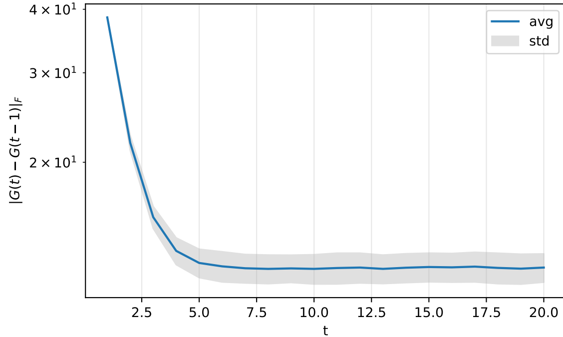
Trajectory-avg step size
