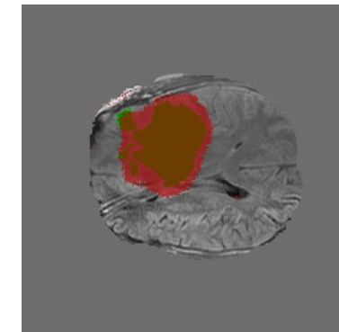
C=64
