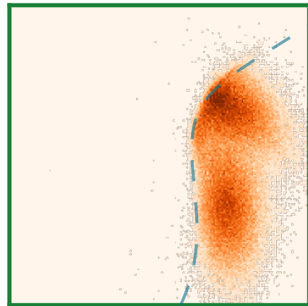
Functa (ours)
