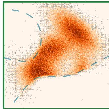
Implicit (ours)
