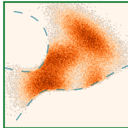
Explicit (ours)
