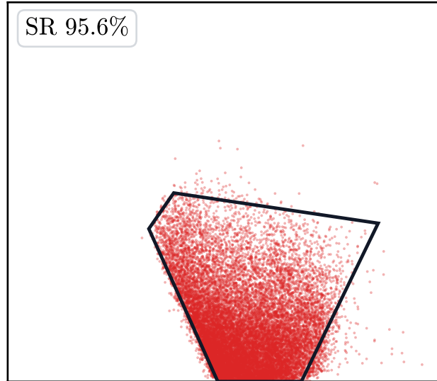
Functa (ours)
