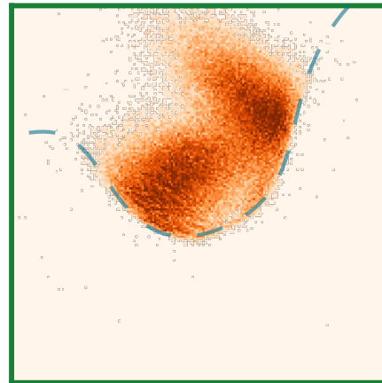
Functa (ours)
