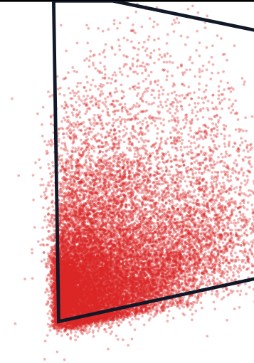
Functa (ours)
