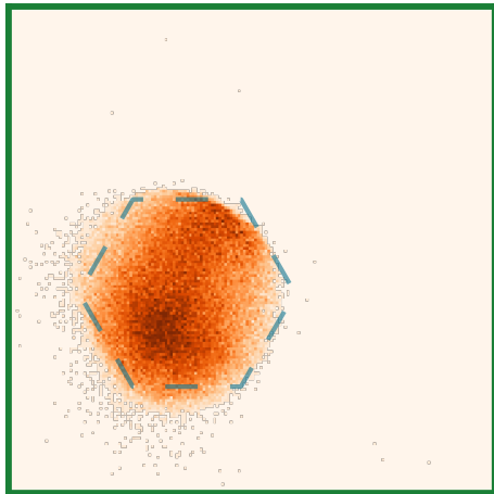
Functa FM
