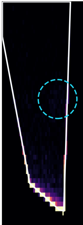
ECI
