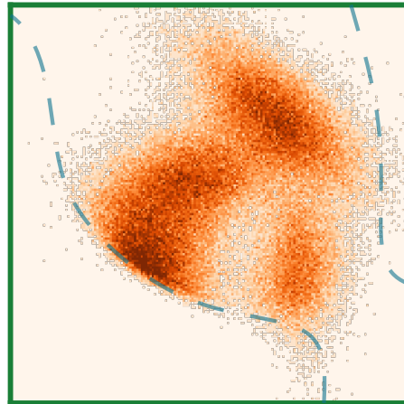
Implicit (ours)
