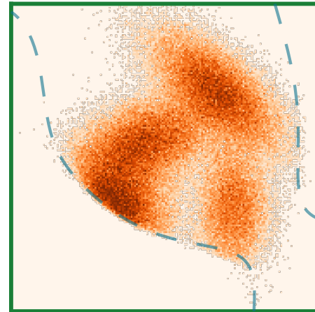
Explicit (ours)
