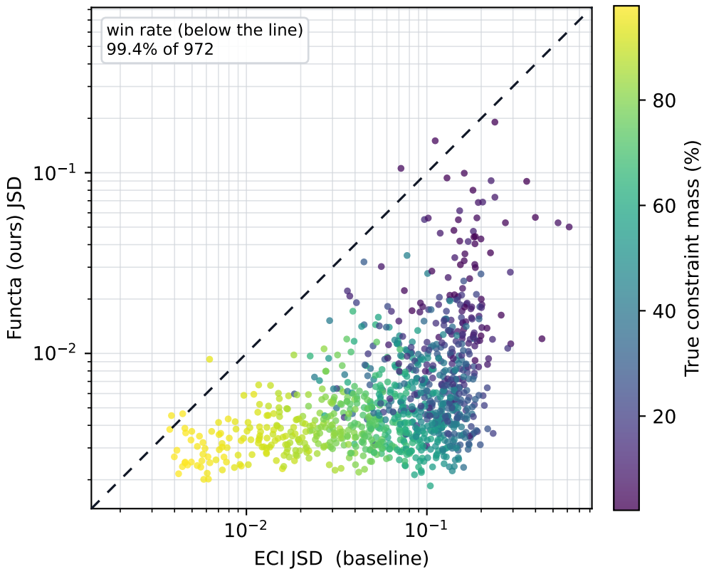
Functa (ours) vs ECI
