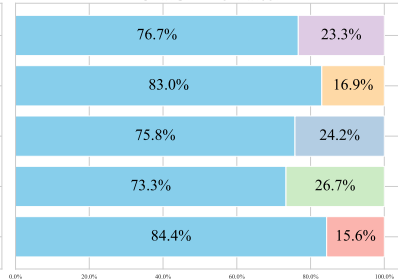
ChatGPT-4o-Latest
