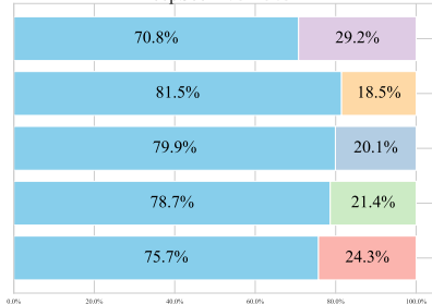
DeepSeek-V3-250324
