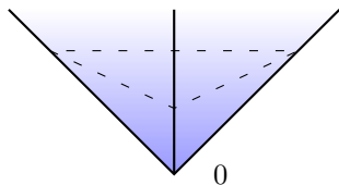
图 14-6: 凸锥与截面
