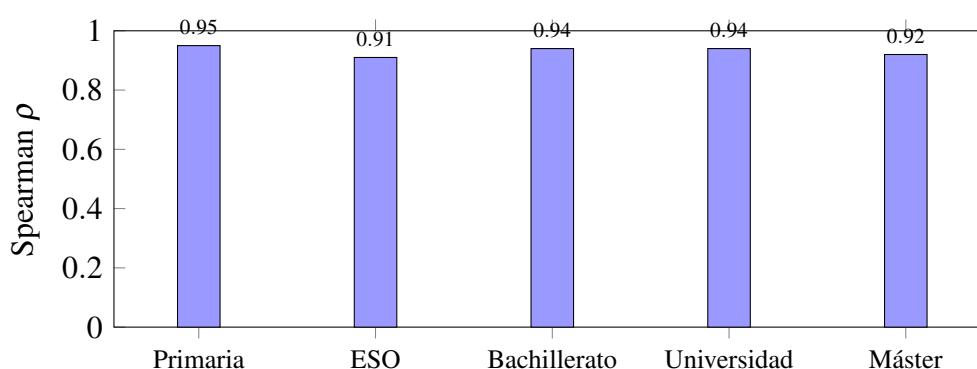
Figura 4.1: Correlación de Spearman por nivel educativo (versión con sinónimos).
