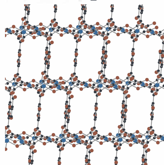
7. DB12-VAGTAA_clean
