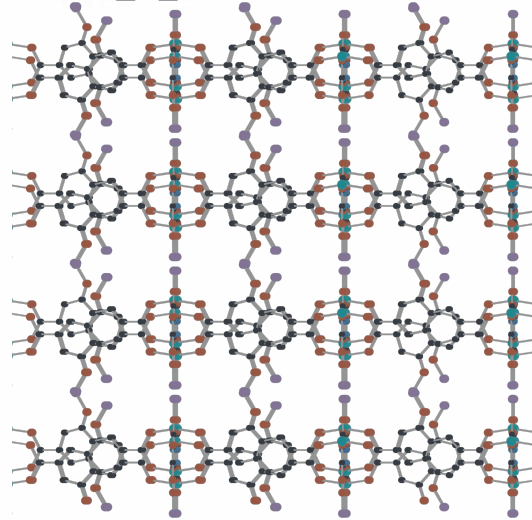
1. DB1-Zn2O8-AZO_irmof8_A_No357
