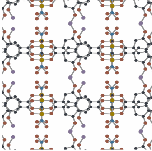
2. DB1-Cu2O8-AZO_A-irmof8_A_No499
