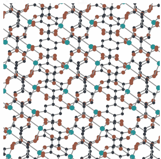
5. DB12-OSAVUA_clean
