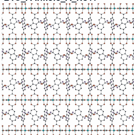
6. DB1-Zn2O8-BTC_A-irmof8_A_No11
