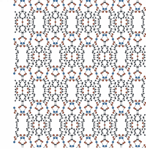
4. DB12-TIXVON_clean
