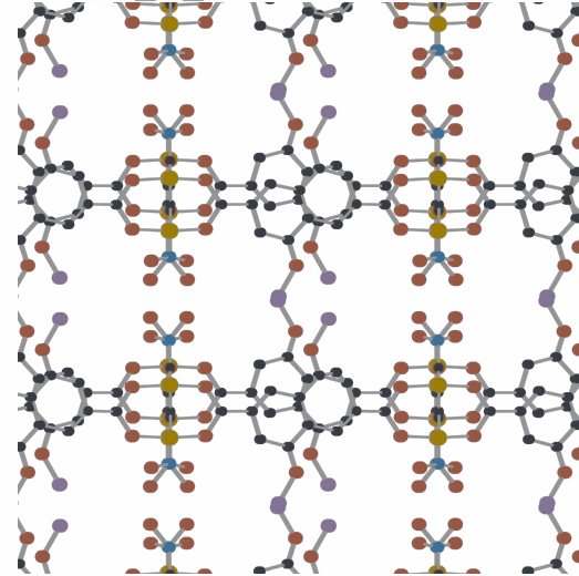
3. DB1-Cu2O8-ADC_A-irmof8_A_No805
