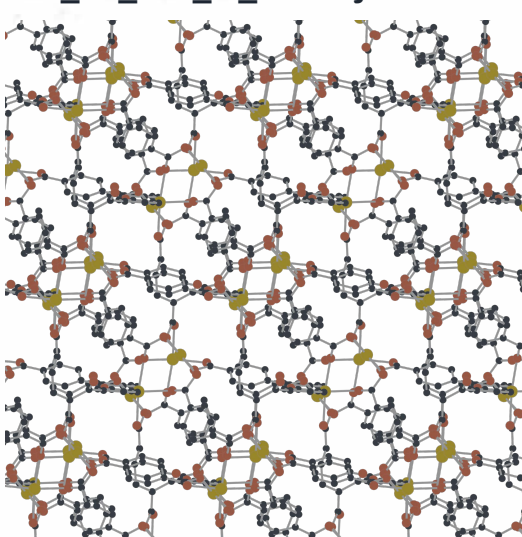
14. DB0-m5_o1_o11_f0_bcu.s ym.34
