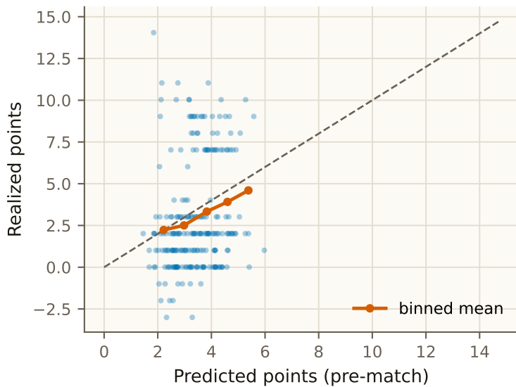
MID (n=1494)
