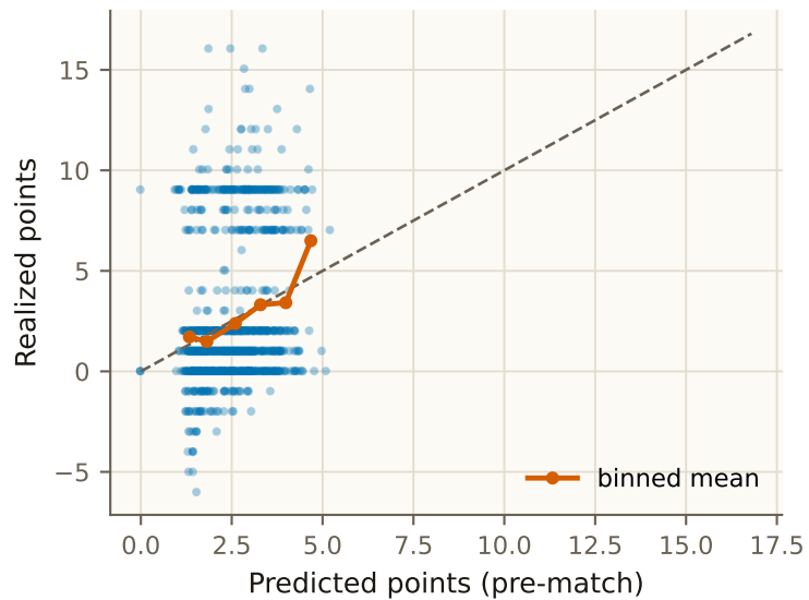
FWD (n=880)
