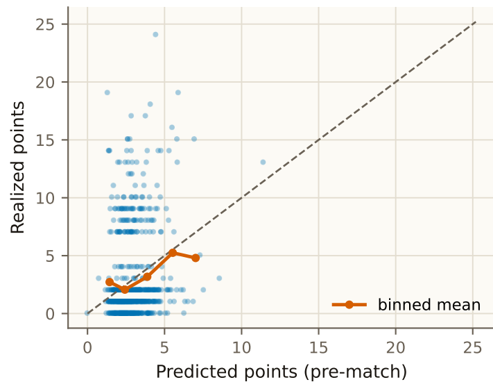
FWD (n=880)
