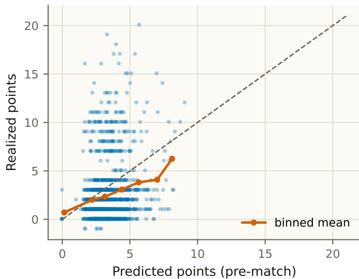
MID (n=1494)
