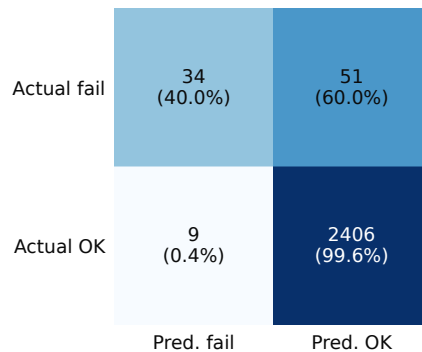
KNN
