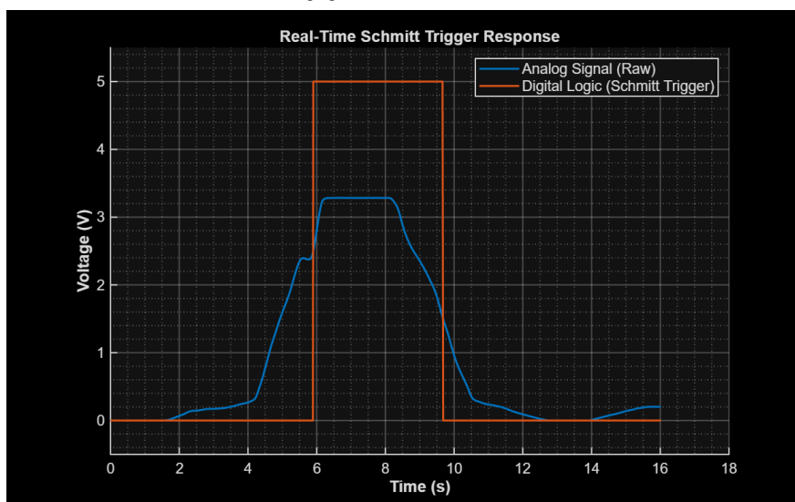
ภาพผลการตอบสนองของวงจร Schmitt Trigger ที่ตั้งค่า Upper Threshold 2.5 V และ Lower Threshold 1.5 V
