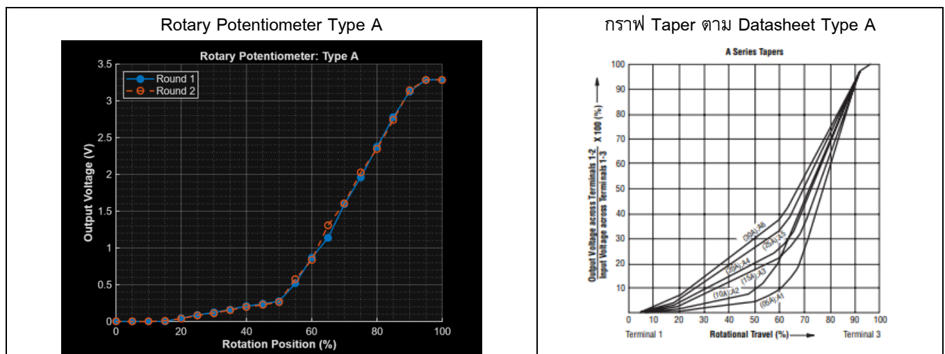
ภาพการเปรียบเทียบการตอบสนองของแรงดันไฟฟ้าของ Rotary Potentiometer ชนิด A ระหว่างผลการทดลองกับกราฟอ้างอิง (Datasheet)
