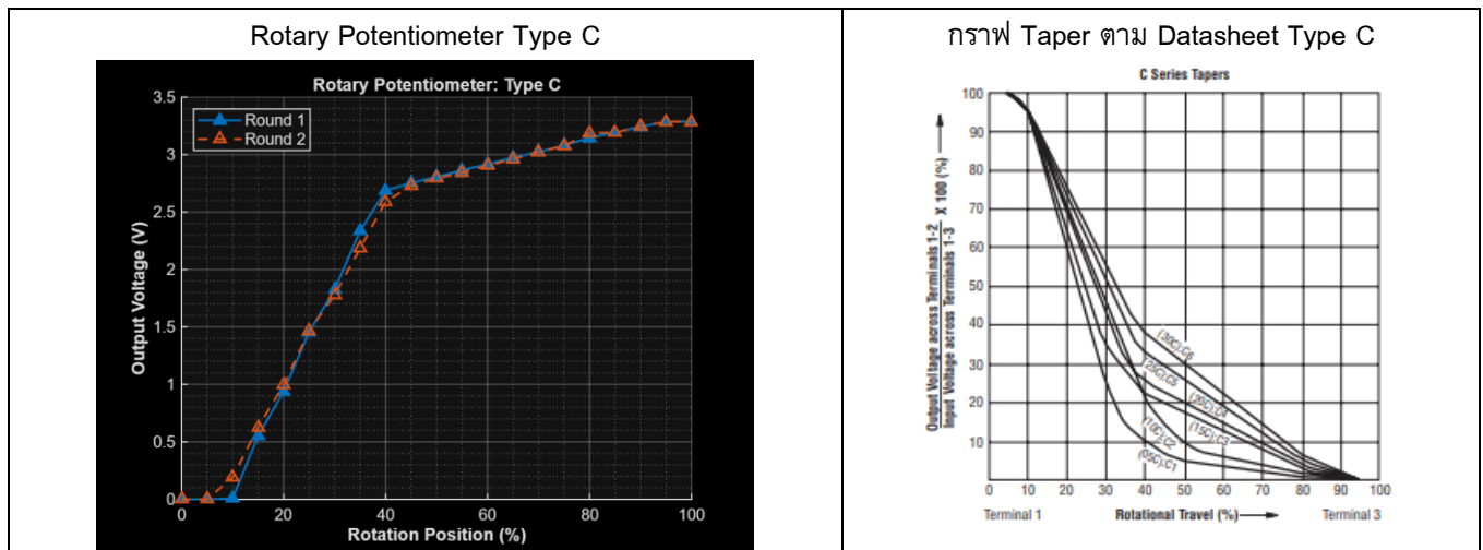
ภาพการเปรียบเทียบการตอบสนองของแรงดันไฟฟ้าของ Rotary Potentiometer ชนิด C ระหว่างผลการทดลองกับกราฟอ้างอิง (Datasheet)
