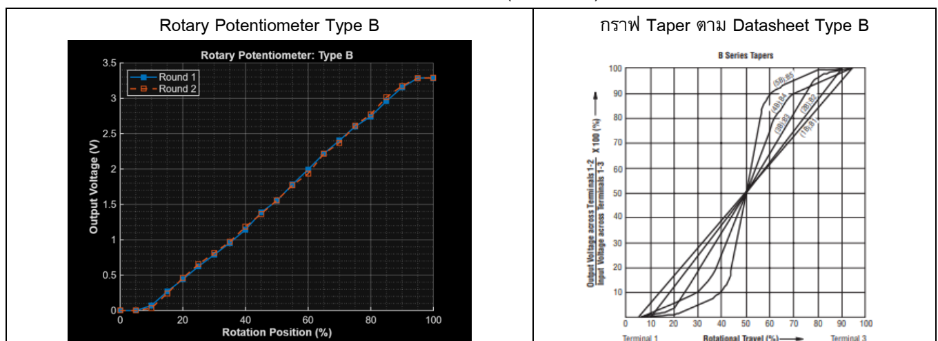
ภาพการเปรียบเทียบการตอบสนองของแรงดันไฟฟ้าของ Rotary Potentiometer ชนิด B ระหว่างผลการทดลองกับกราฟอ้างอิง (Datasheet)
