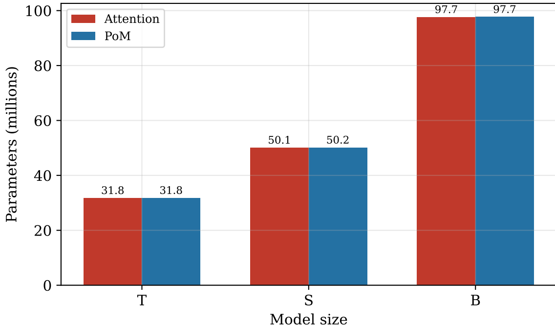
Matched parameter budget (PoM adds < 0.1%)
