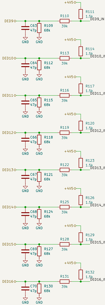
D9–D16 (J3)
