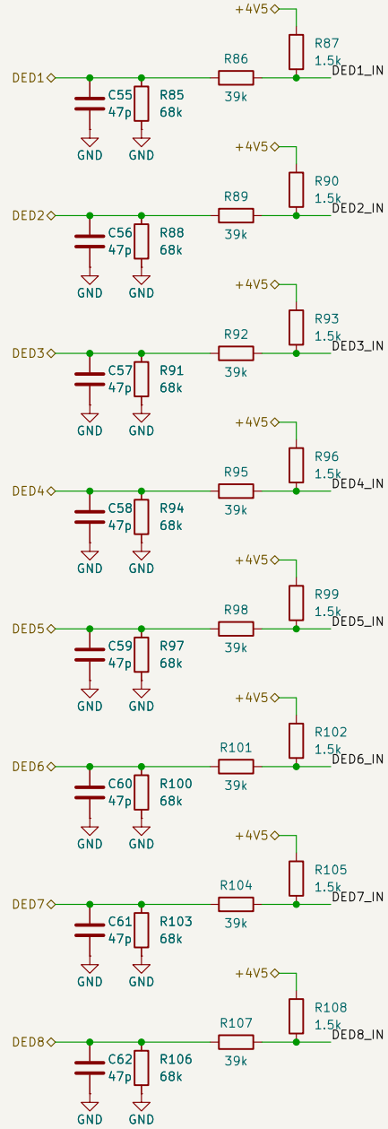
D1–D8 (J2)
