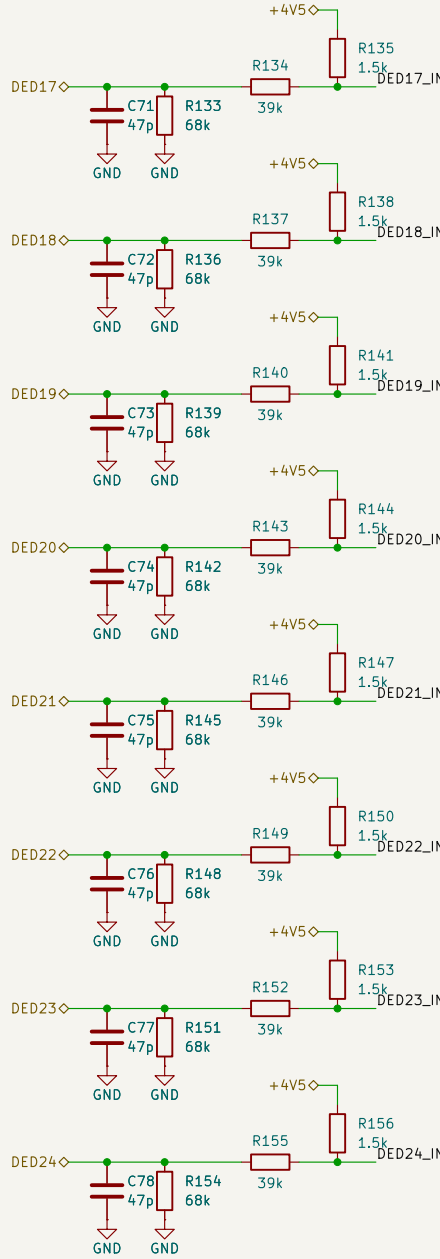
D17–D24 (J13)
