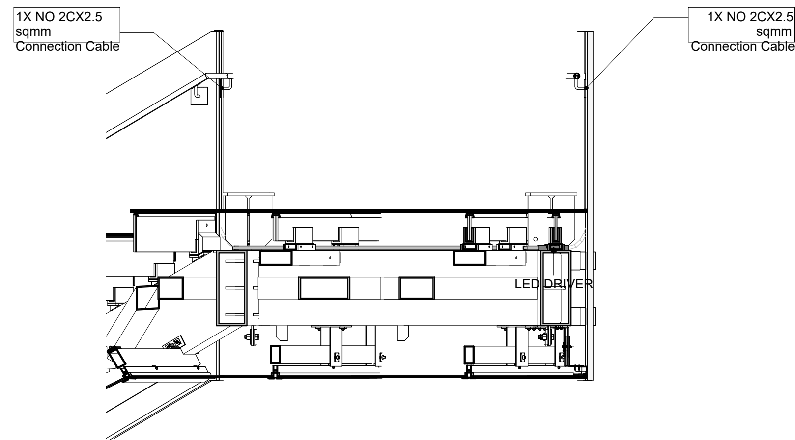
02_Level 02 27500.00n +27.500 m
