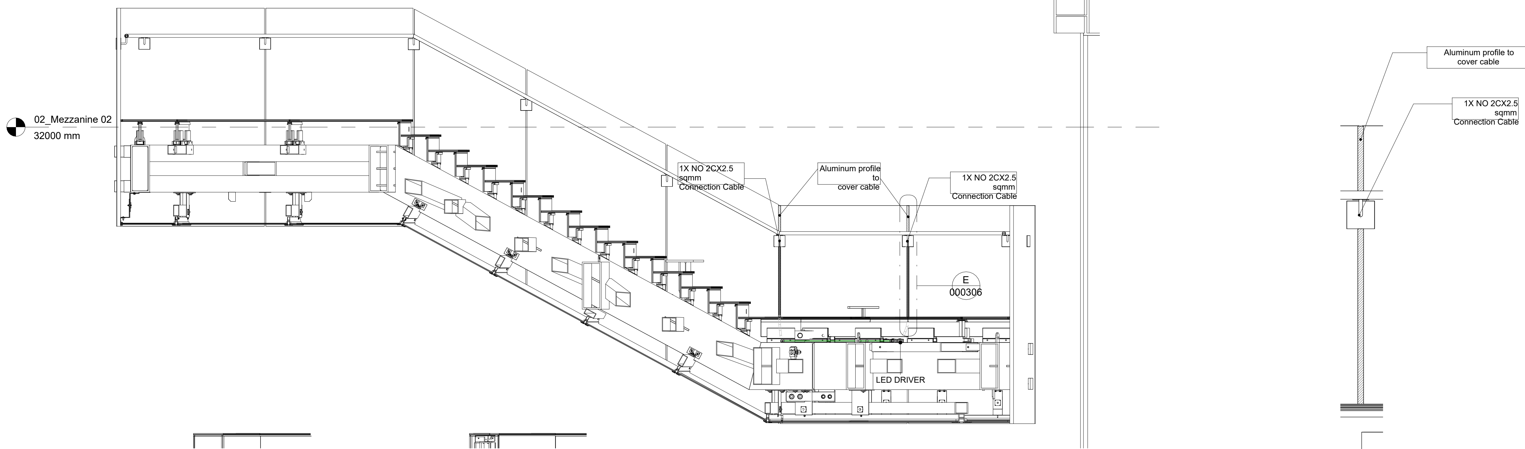
B STAIR AU - SECTION B 1 : 25
