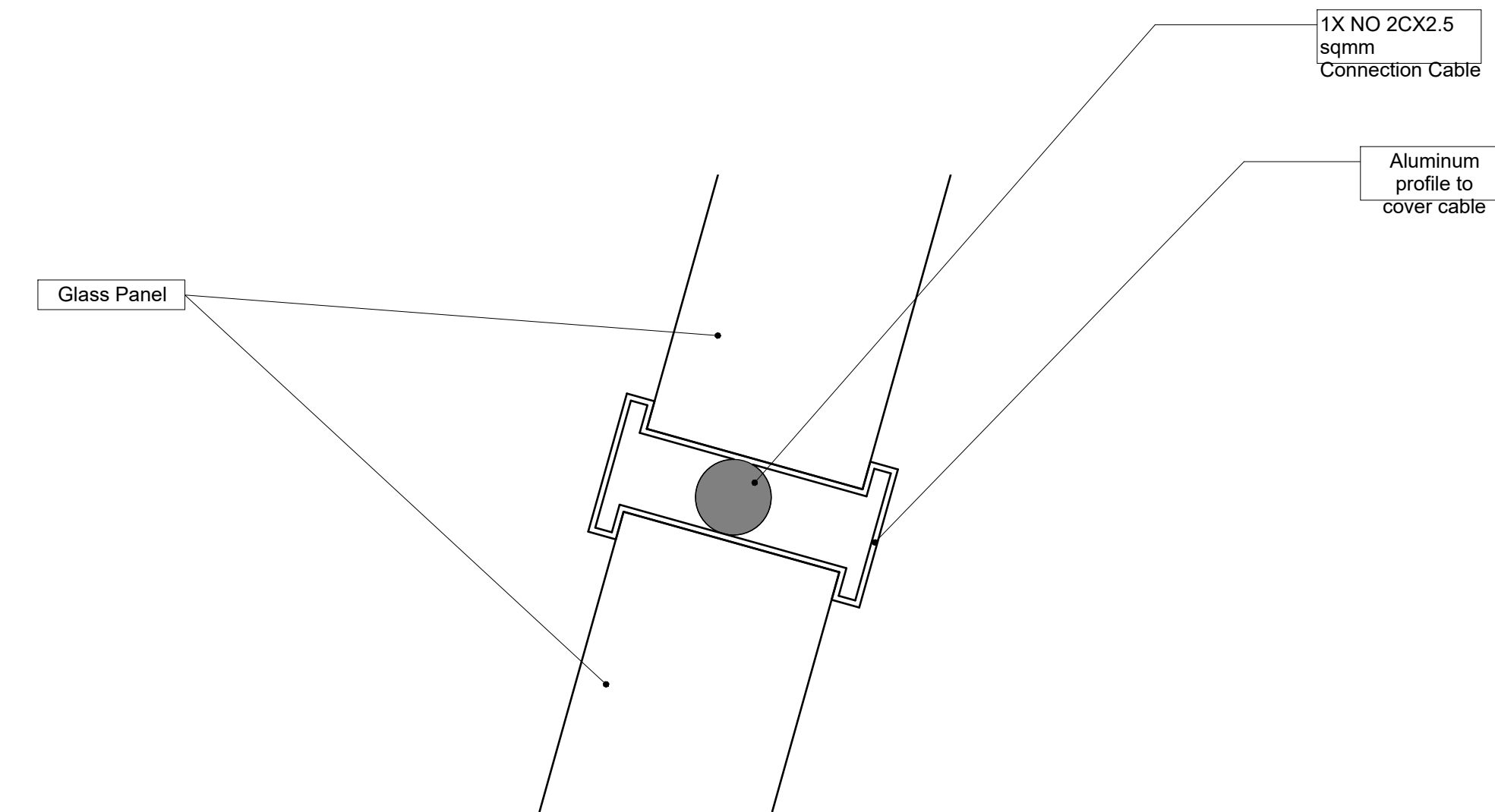
D STAIR AU - WIRE CONNECTION 1 : 1
