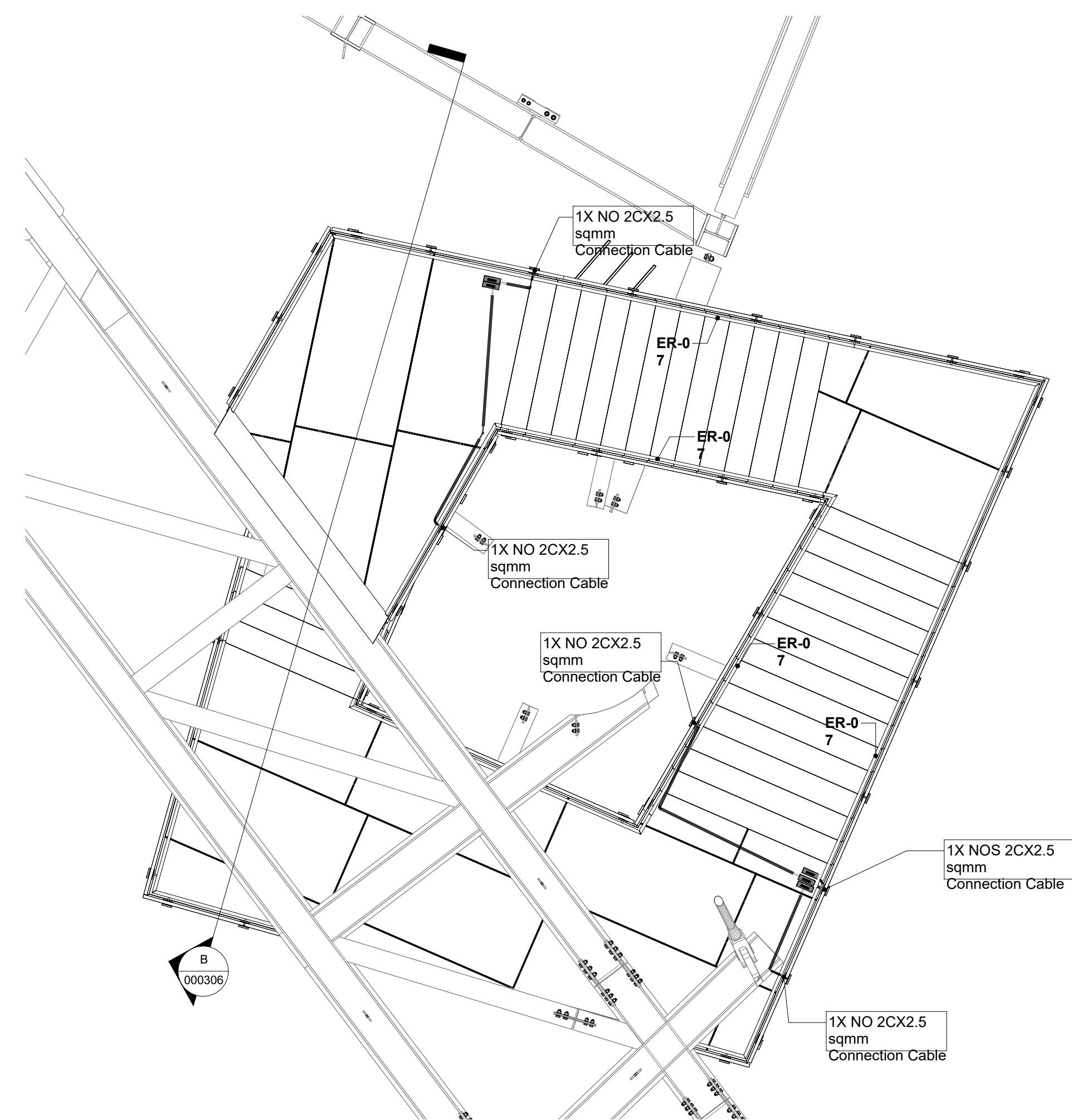
2 STAIR AU MEZZANINE 02 1 : 50
