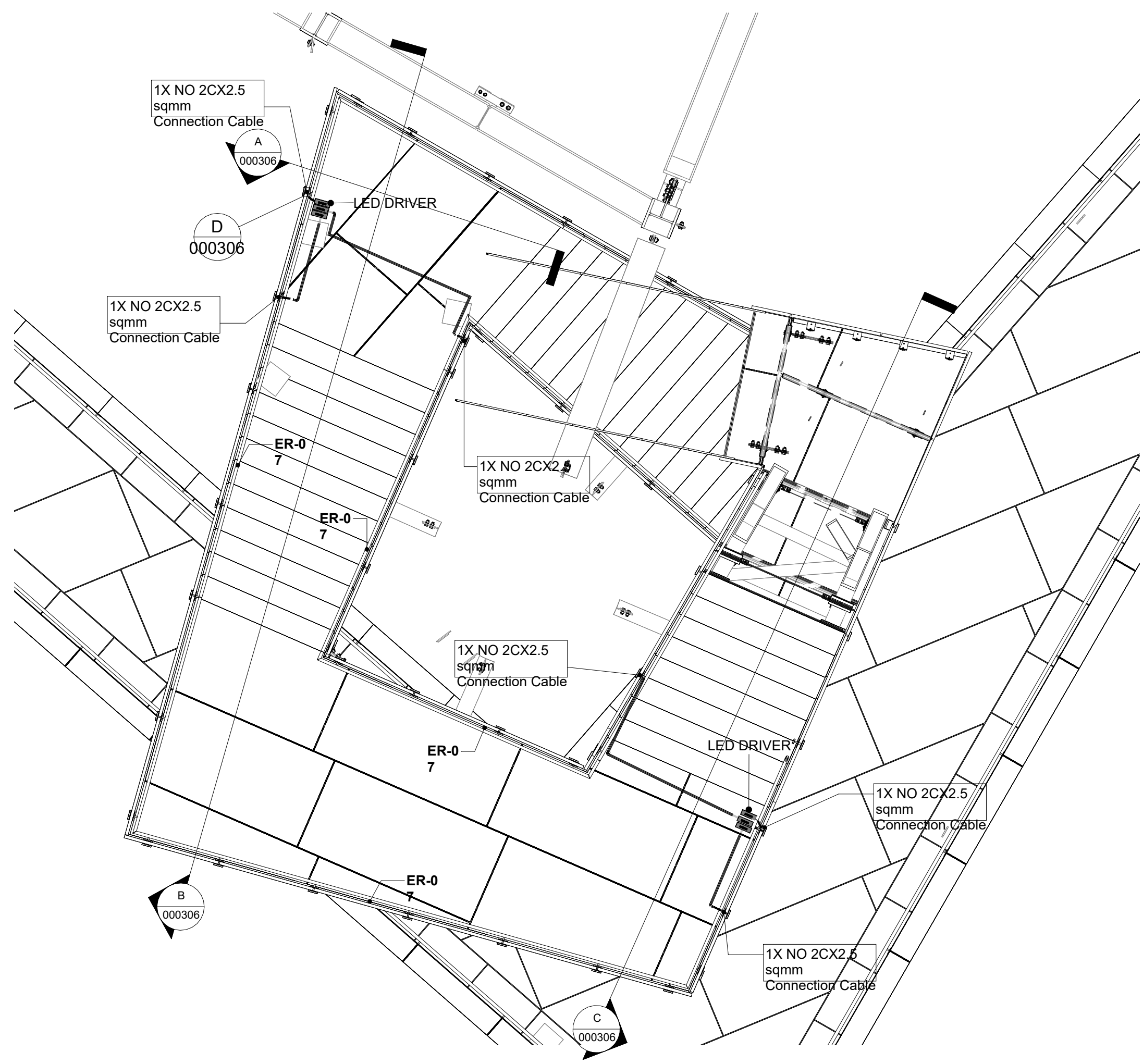
1 STAIR AU Level 02 1 : 50
