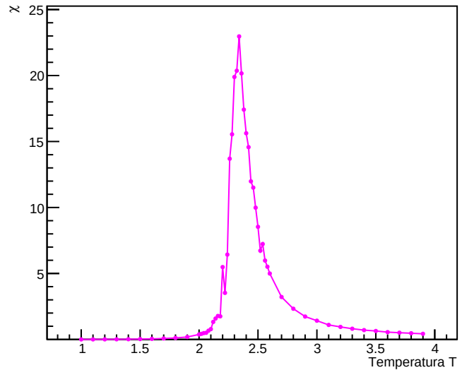
Suscettività Magnetica per spin
