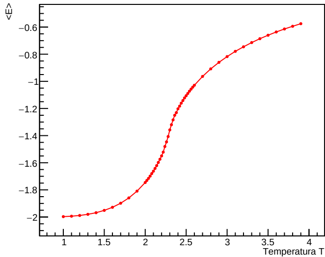
Energia Media per spin
