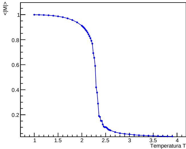
Magnetizzazione Media assoluta per spin
