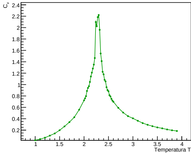
Calore Specifico per spin
