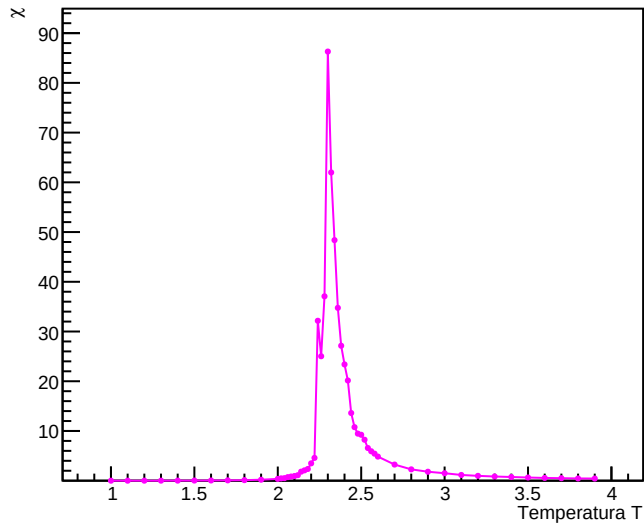
Suscettività Magnetica per spin
