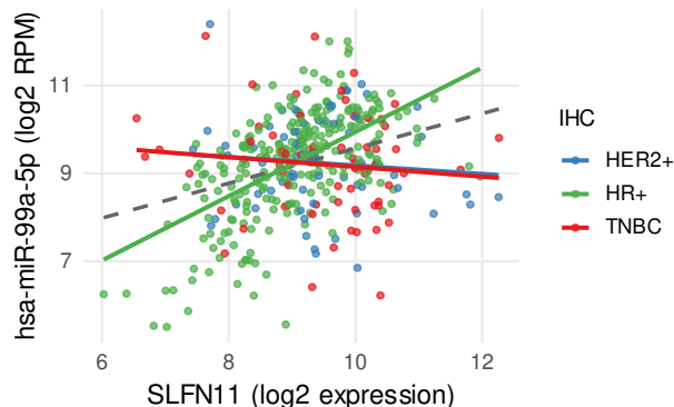
D. IHC exemplar: SLFN11 x hsa-miR-99a-5p
