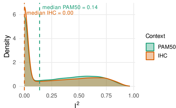
D. IHC exemplar: SLFN11 x hsa-miR-99a-5p
