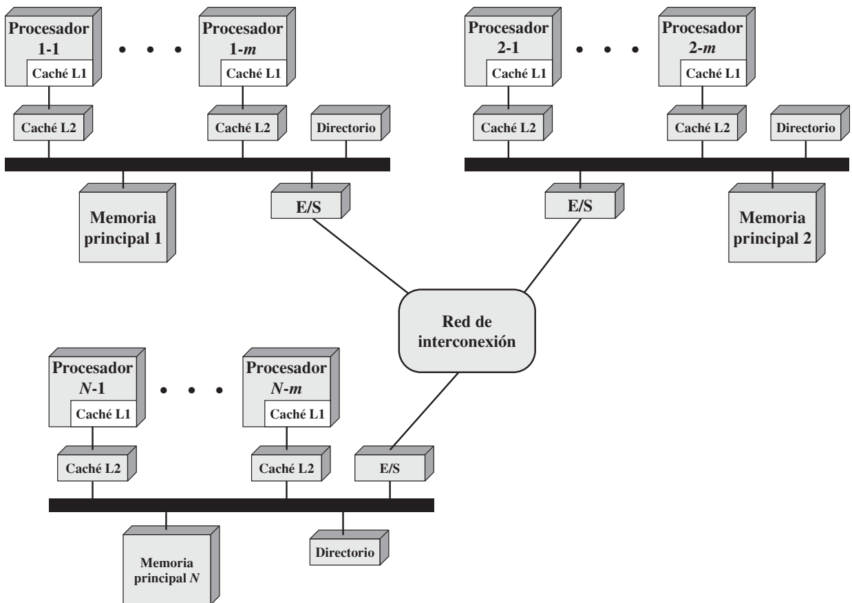
Figura 18.12. Organización CC-NUMA.
