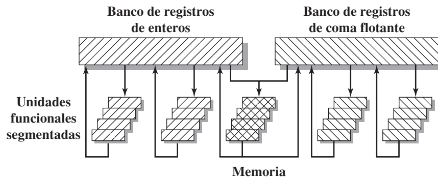
Figura 14.1. Organización superescalar general [COME95].
