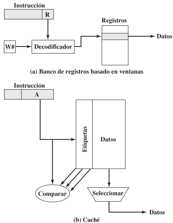
Figura 13.3. Referencia a un dato escalar.
