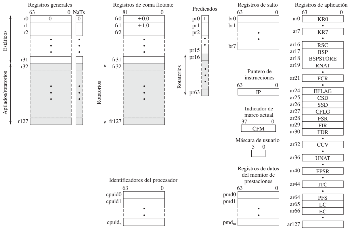
Figura 15.7. Conjunto de registros de aplicación de IA-64.
