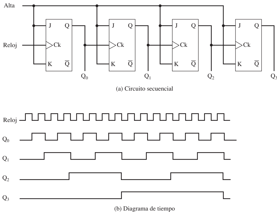
Figura B.32. Contador ondulado.
