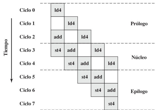
Figura 15.6. Ejemplo de segmentación software.
