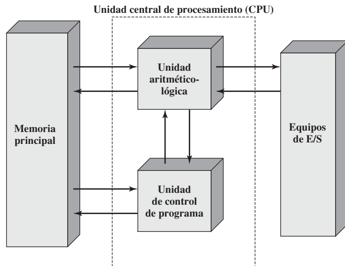
Figura 2.1. Estructura del computador IAS.
