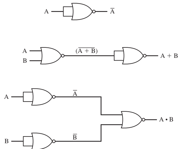
Figura B.3. Uso de las puertas NOR.
