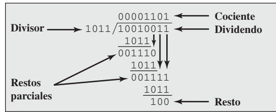
Figura 9.15. División de enteros binarios sin signo.
