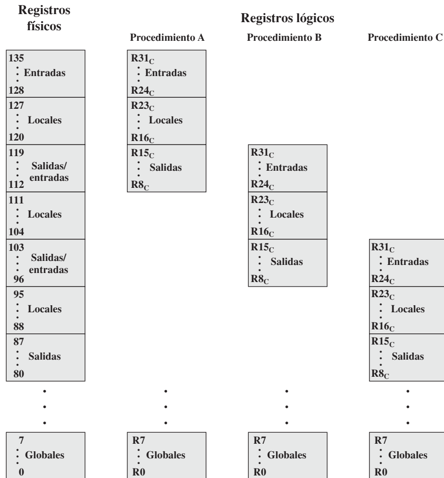
Figura 13.11. Disposición de las ventanas de registros del SPARC para tres procedimientos.
