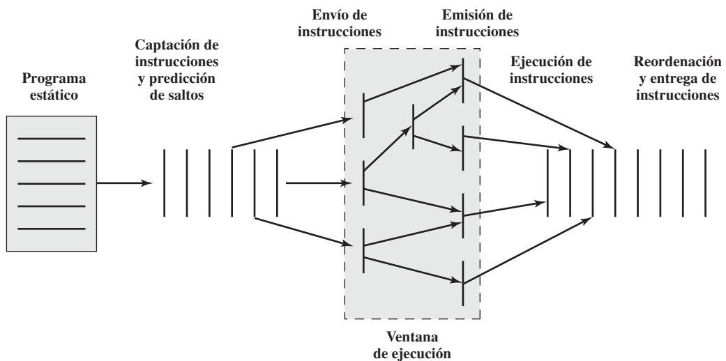
Figura 14.6. Representación conceptual del procesamiento superescalar [SMIT95].
