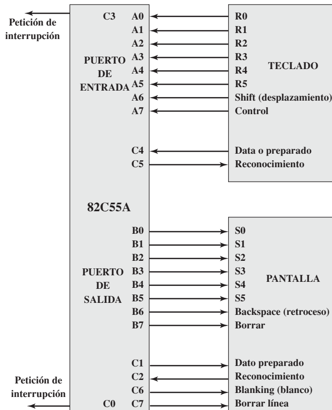
Figura 7.10. Interfaz teclado/pantalla en el 82C55A.
