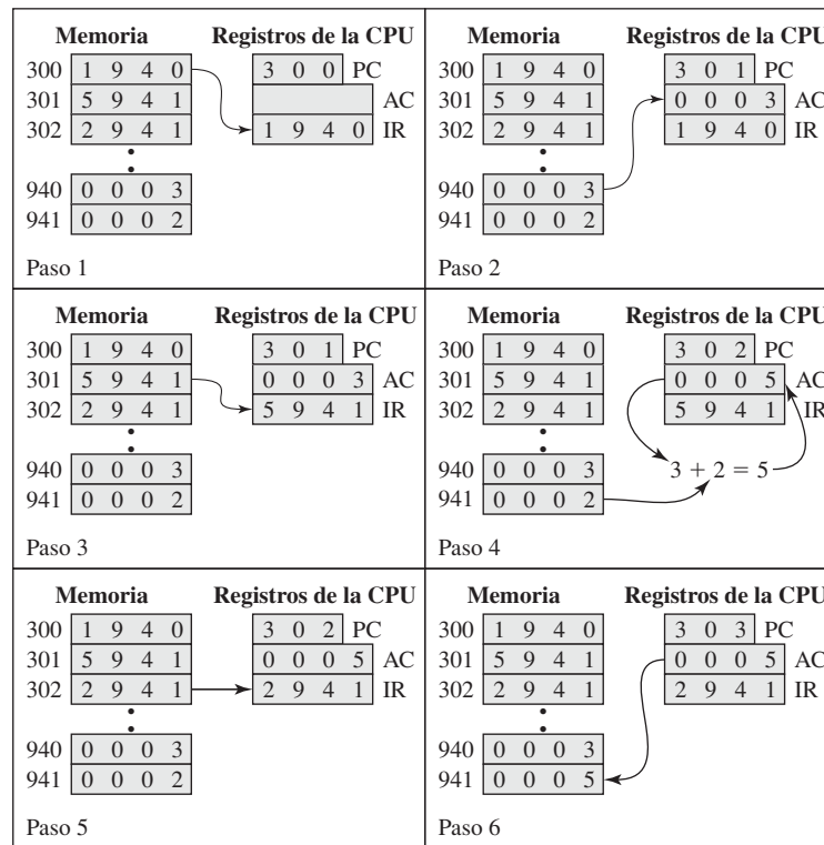
Figura 3.5. Ejemplo de ejecución de un programa (contenidos de la memoria y de los registros en hexadecimal).
