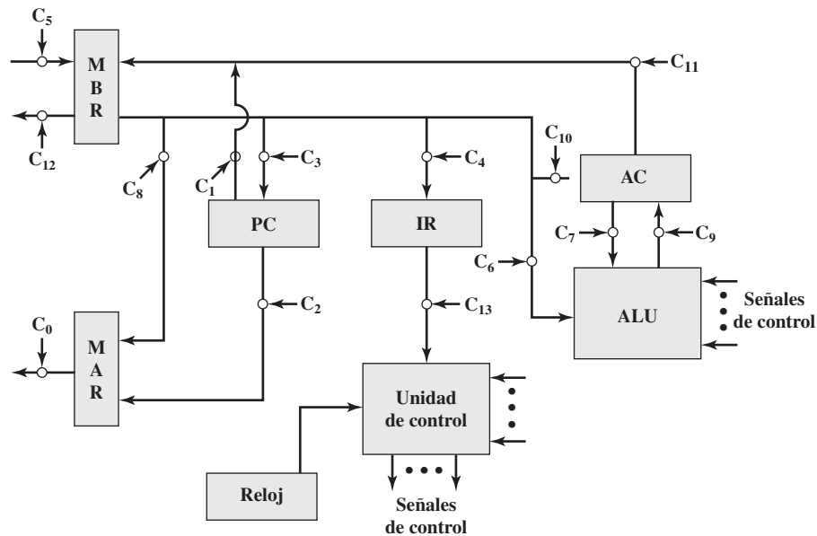
Figura 16.5. Caminos de datos y señales de control.
