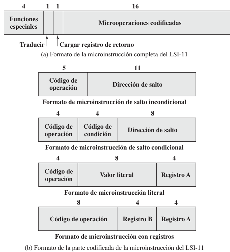
Figura 17.15. Formato de microinstrucción del LSI-11.
