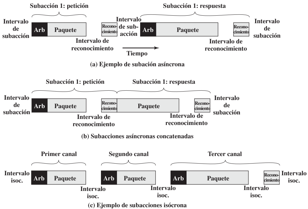
Figura 7.19. Subacciones FireWire.
