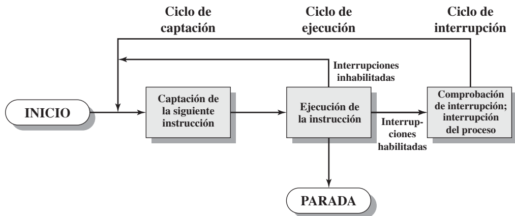
Figura 3.9. Ciclo de instrucción con interrupciones.
