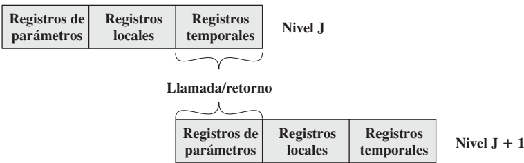
Figura 13.1. Ventanas de registro solapadas.
