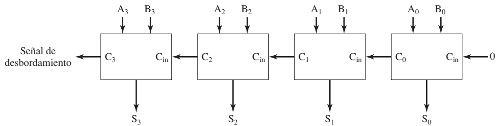
Figura B.21. Sumador de cuatro bits.
