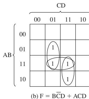
Figura B.9. Grupos solapados.
