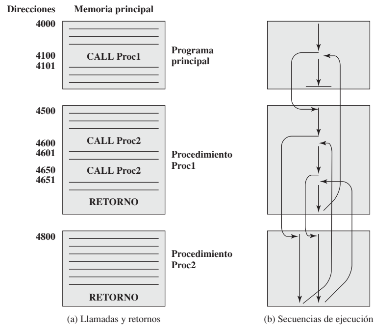
Figura 10.7. Procedimientos anidados.
