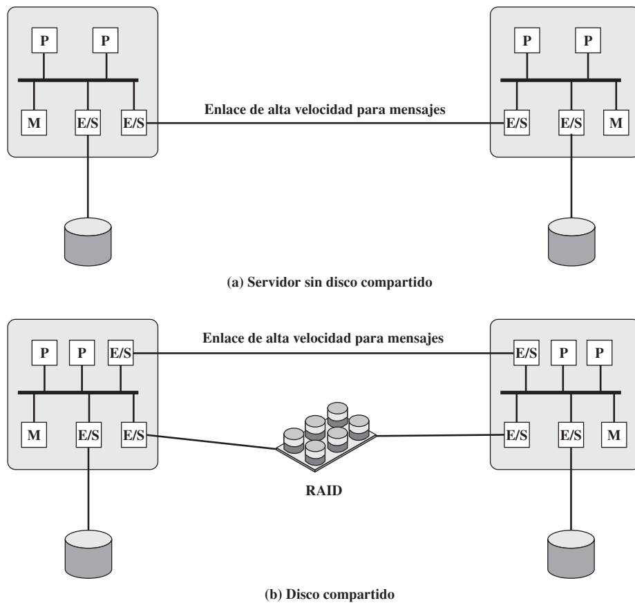
Figura 18.10. Configuraciones de cluster .
