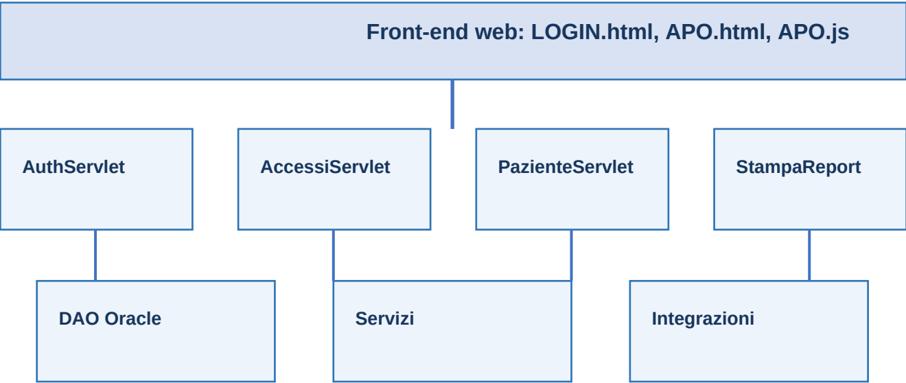
Figura - Architettura logica AmbMMG
