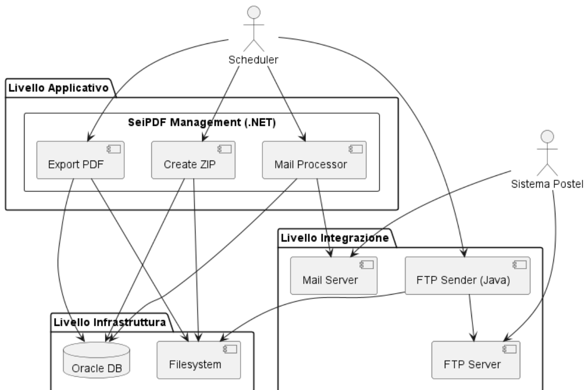
Immagine 2 – Architettura a livelli
