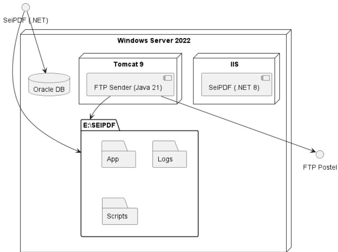
Immagine 3 – Architettura fisica
