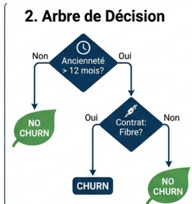
FIGURE 4.2 – Principe de l'Arbre de Décision
