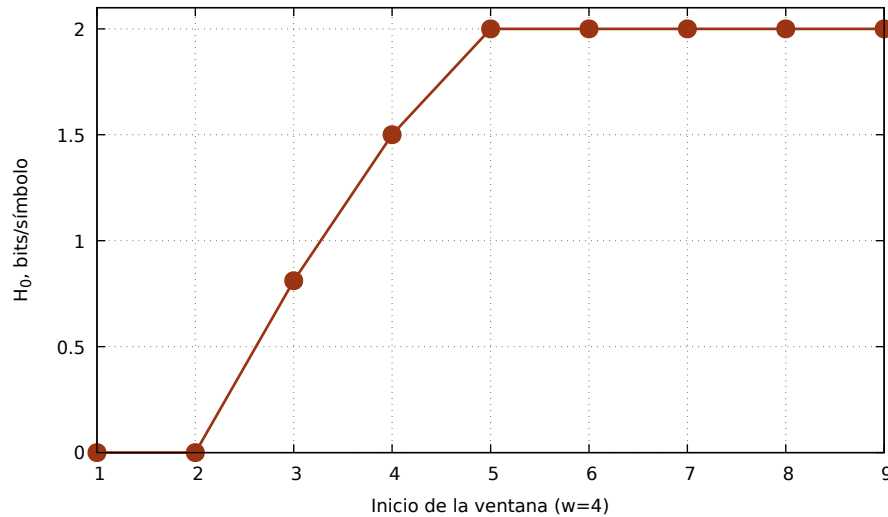
Figure 1.4: Perfil reproducible de AAAAACGTACGT con ancho cuatro. Activo original TC07-F03, generado por make_figures.sh windows desde TC07-F03-windows.tsv . Los puntos son ventanas discretas; la línea solo guía su lectura. Texto alternativo: nueve puntos que toman sucesivamente los valores 0, 0, 0,811278, 1,5 y después cinco veces 2.
