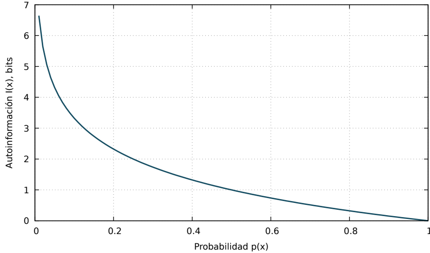
Figure 1.1: Autoinformación frente a probabilidad. En el dominio representado, -\log_2 p(x) crece rápidamente al disminuir p(x) . Activo original TC07-F01, generado por make_figures.sh selfinfo desde TC07-F01-selfinfo.tsv. Texto alternativo: curva decreciente desde valores altos para probabilidades pequeñas hasta cero cuando la probabilidad es uno.
