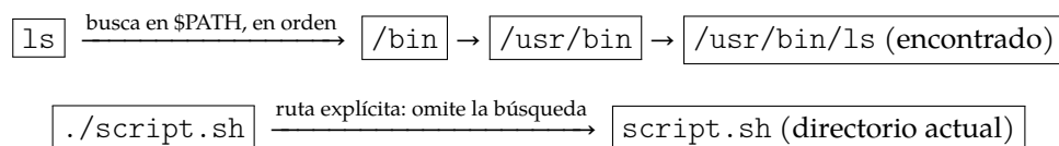
Figura 4: Arriba, el nombre ls se busca en cada directorio de $PATH hasta encontrar /usr/bin/ls ; abajo, la ruta explícita ./script.sh evita esa búsqueda y usa el fichero del directorio actual. Figura original.
