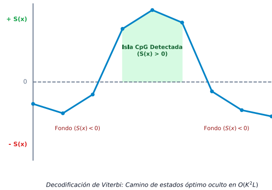
B) Perfil de Log-Odds Ratio: S(x) = \log_2 \frac{P(x|+)}{P(x|-)}
