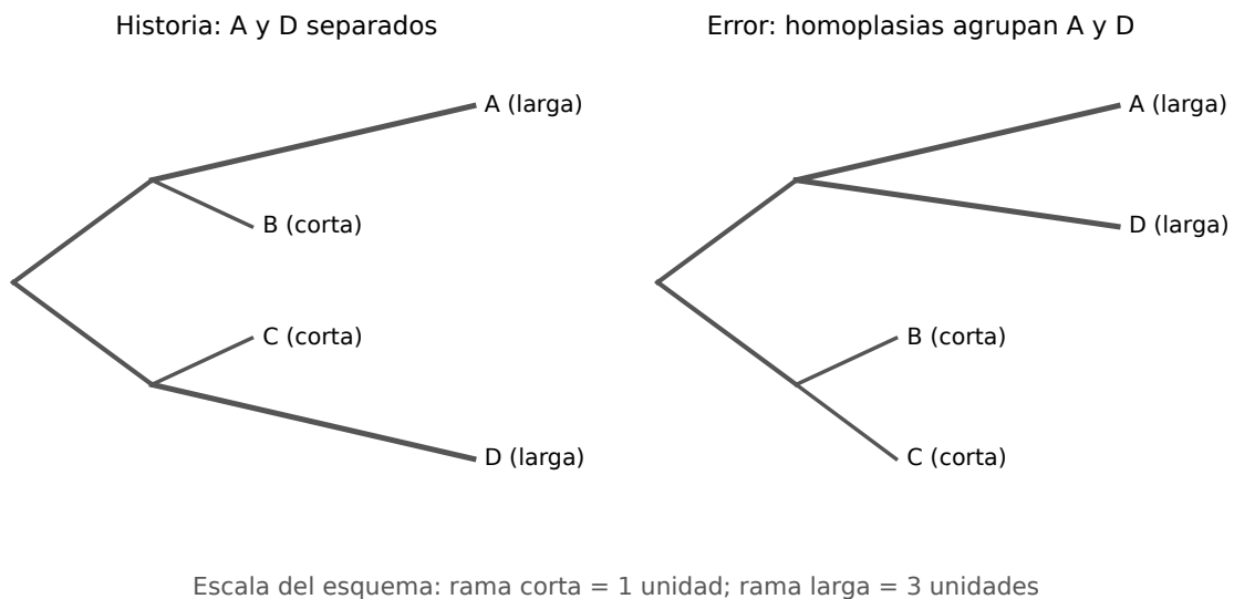
Figura 10: Esquema conceptual de atracción de ramas largas. No representa una simulación empírica ni afirma que toda rama larga sea artefactual.
