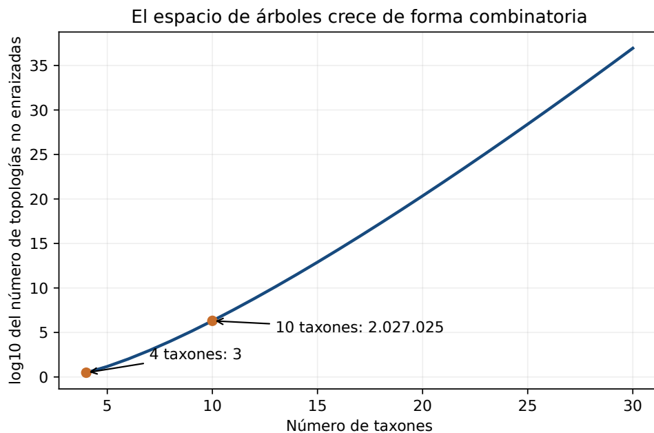
Figura 8: Crecimiento del número de topologías bifurcantes no enraizadas. El eje vertical usa logaritmo decimal para que la curva pueda representarse.
