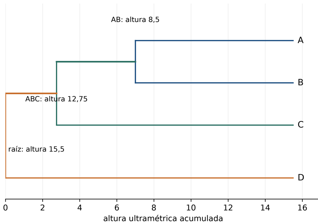
Figura 7: Dendrograma UPGMA reconstruido a partir de la matriz de cuatro taxones. Todas las puntas quedan a altura 15,5.
