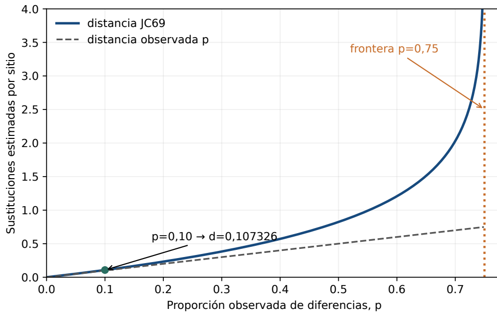
Figura 6: Distancia observada y corrección JC69. La divergencia cerca de p = 0,75 señala la pérdida de información bajo el modelo.
