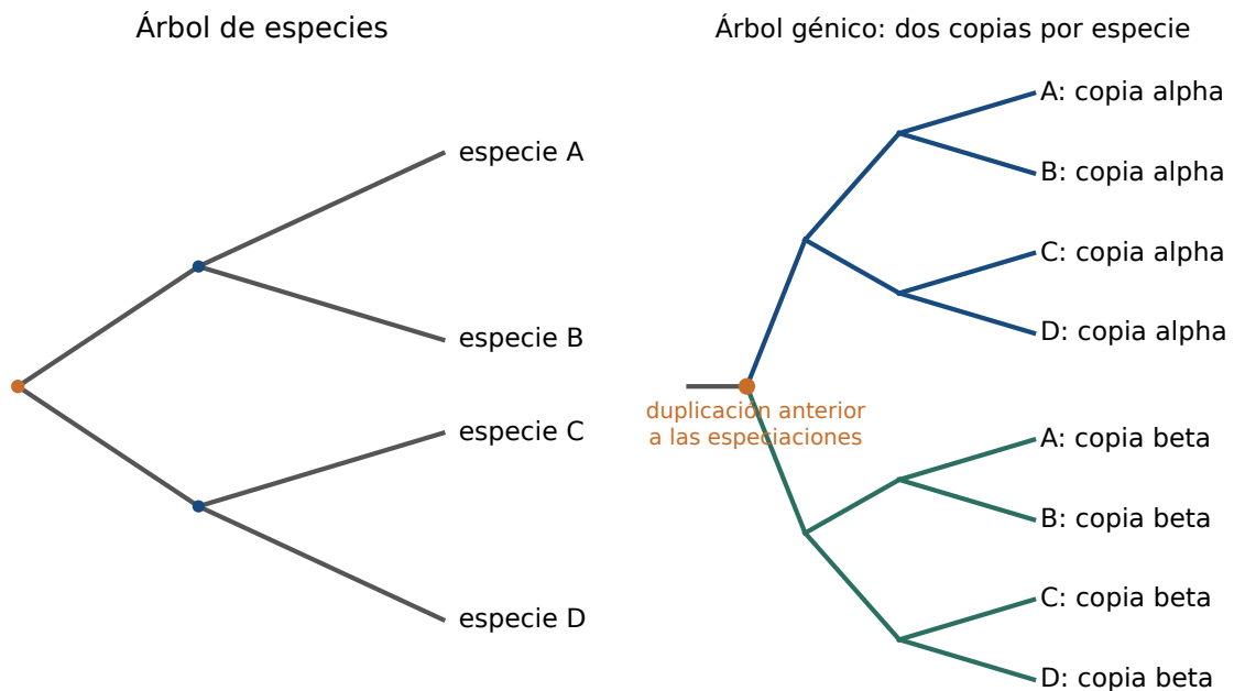
Figura 4: Contraste elemental entre un árbol de especies y un árbol génico afectado por una duplicación anterior a la especiación.
