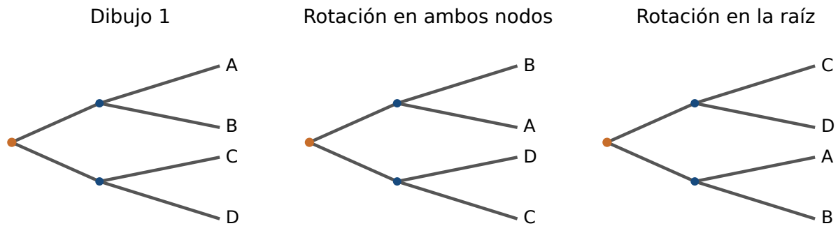
Figura 2: Tres representaciones de la misma topología enraizada. En todos los paneles permanecen los clados {A,B} y {C,D}.
