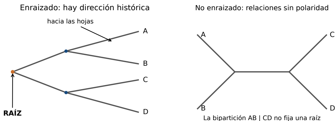
Figura 3: Un árbol enraizado contiene polaridad histórica; el árbol no enraizado solo fija la bipartición mostrada.
