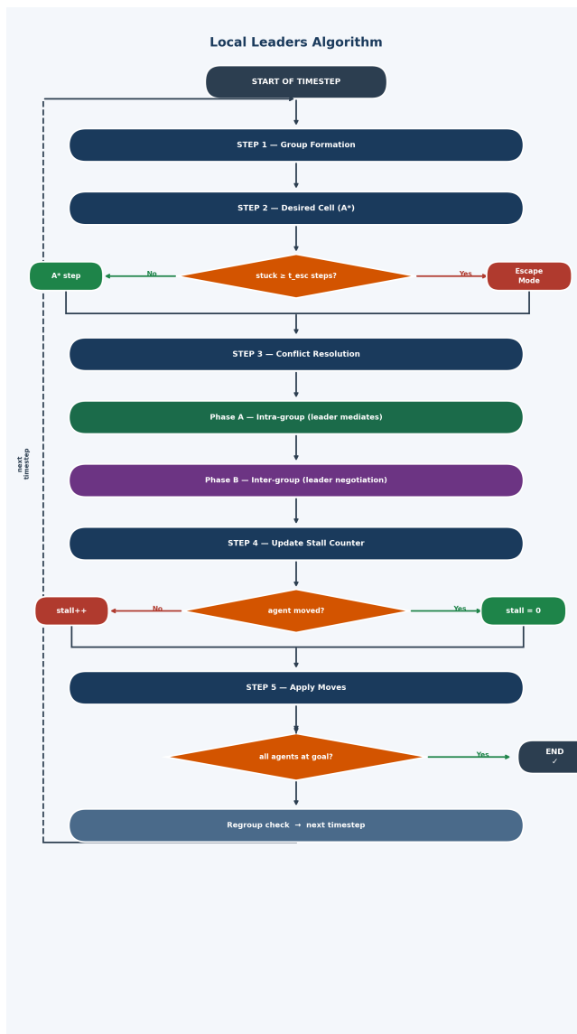
Slika 1: Diagram poteka algoritma Local Leaders: dinamično oblikovanje skupin, določitev vodje, A* načrtovanje in dvofazna razrešitev konfliktov (znotrajskupinska posredovanost vodje, nato medskupinsko pogajanje vodij).
